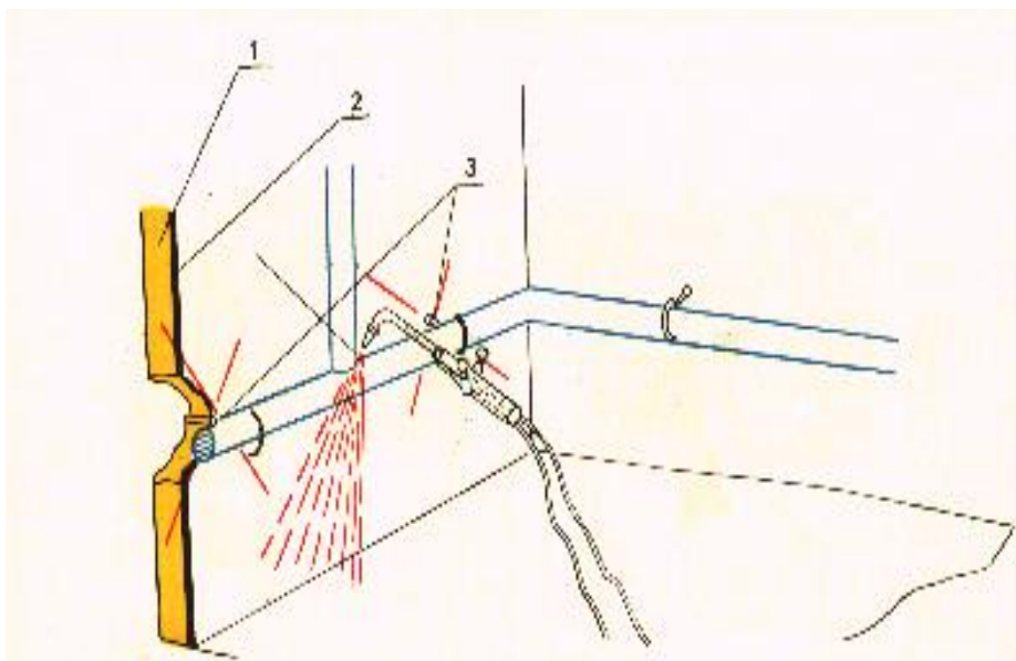
Rys.5. Elementy instalacji rozgrzewające się przy spawaniu od płomienia lub na skutek przewodnictwa cieplnego, stykające się z materiałami palnymi należy zdemontować lub skutecznie chłodzić: 1-palna ścianka, 2-niepalna wykładzina, 3-haki podtrzymujące instalację.
