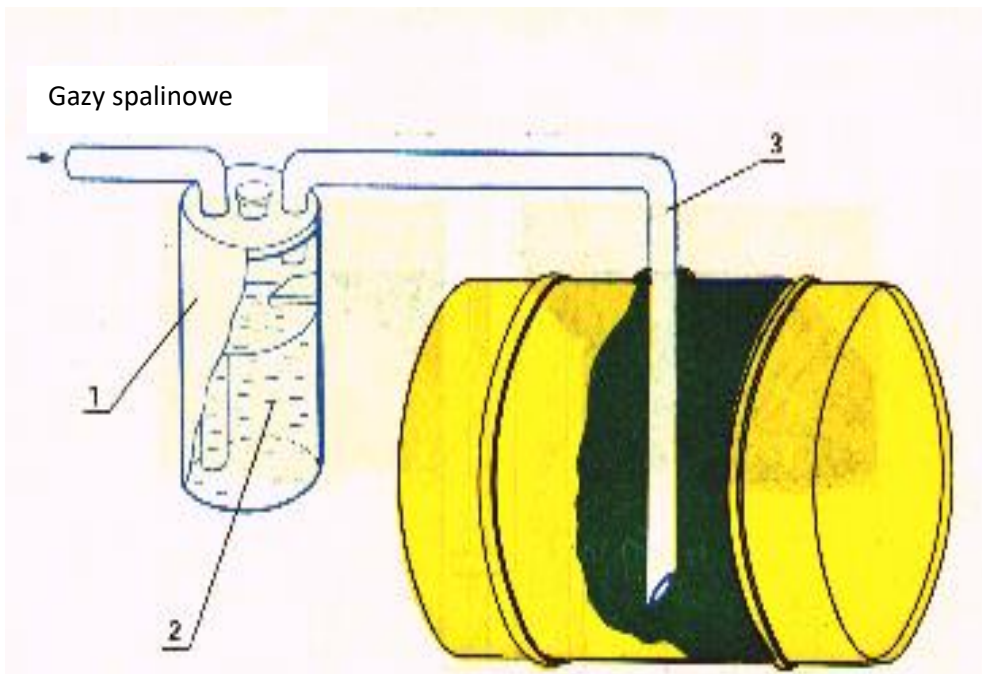
Rys.7. Ciężkie lub spawane pojemniki mogące zawierać gazy lub pary palnych cieczy należy przed przystąpieniem do prac wypełnić gazem obojętnym np. gazami spalinowymi poprzez urządzenie do wylapywania iskier: 1-urządzenie do wylapywania iskier, 2-woda, 3-przewód.
