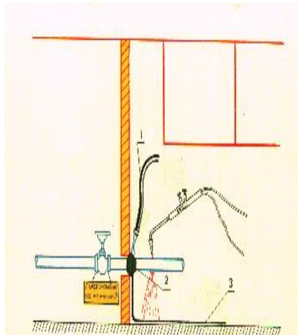
Rys.2. Spawane przewody, części maszyn i urządzeń oraz elementy konstrukcji budowlanych stykające się z materiałami palnymi lub przebiegające w pobliżu nich należy skutecznie chłodzić: 1-przewód donrowadzających wodę. 2-zwoje sznura z materiału
